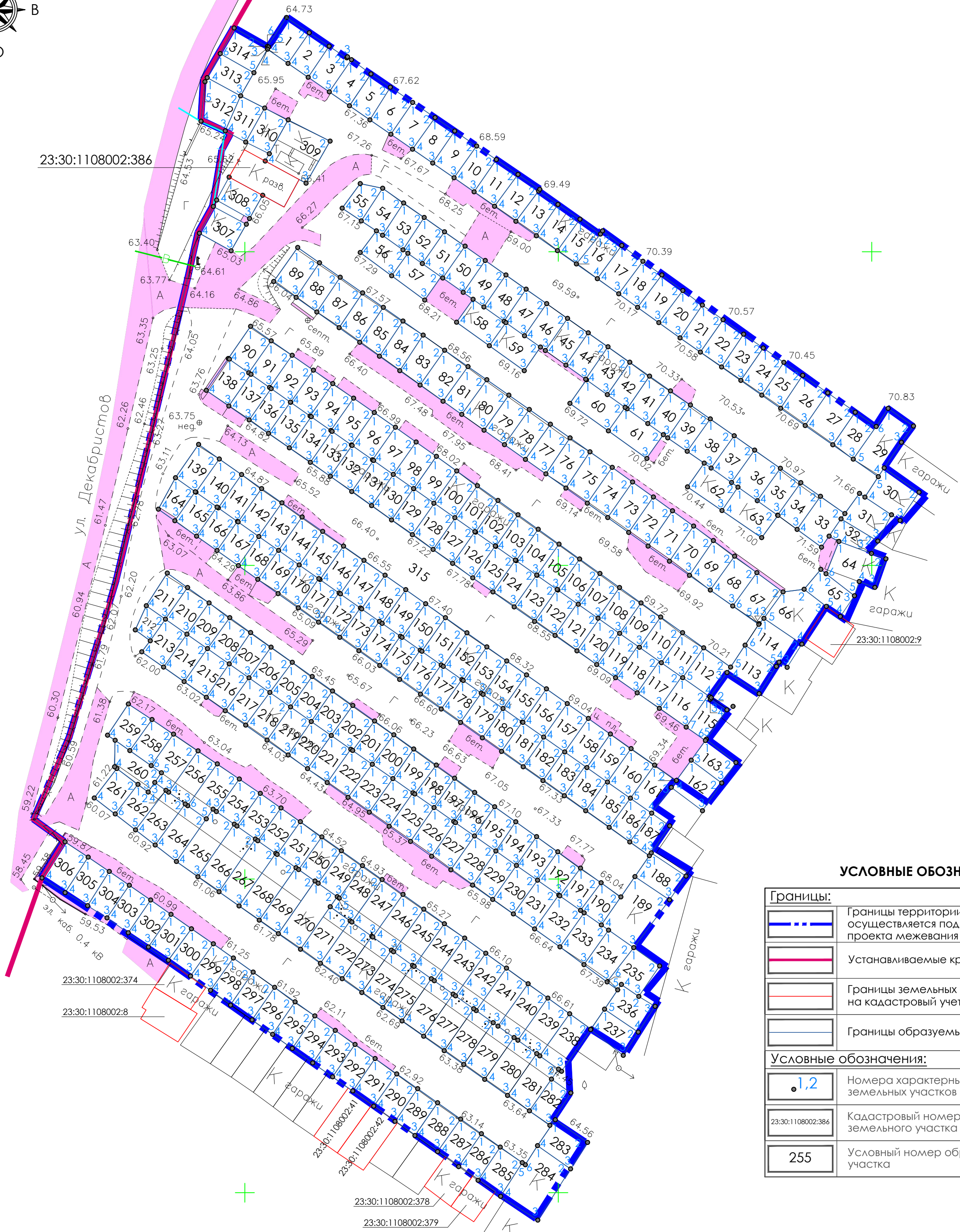
Чертеж межевания территории. М 1:500
