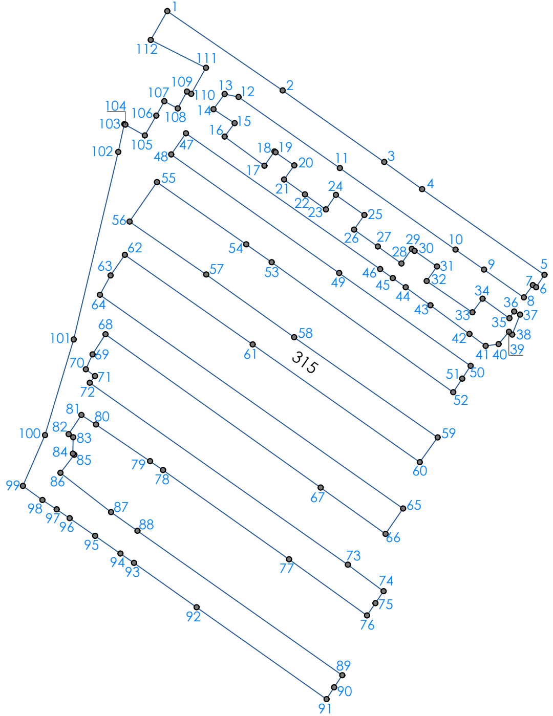
Фрагмент чертежа межевания территории. Контур ЗУ с условным номером :ЗУ315. М 1:1000
